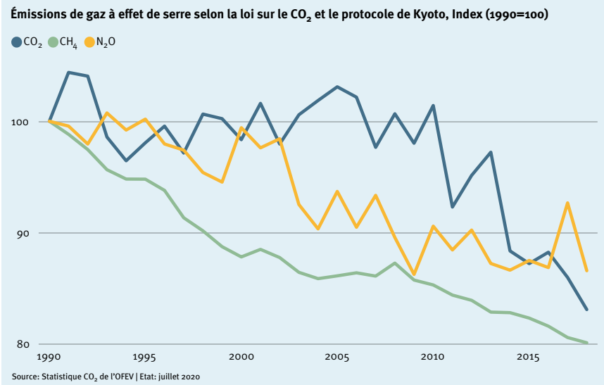
Source: Statistique CO 2 de l'OFEV | Etat: juillet 2020
