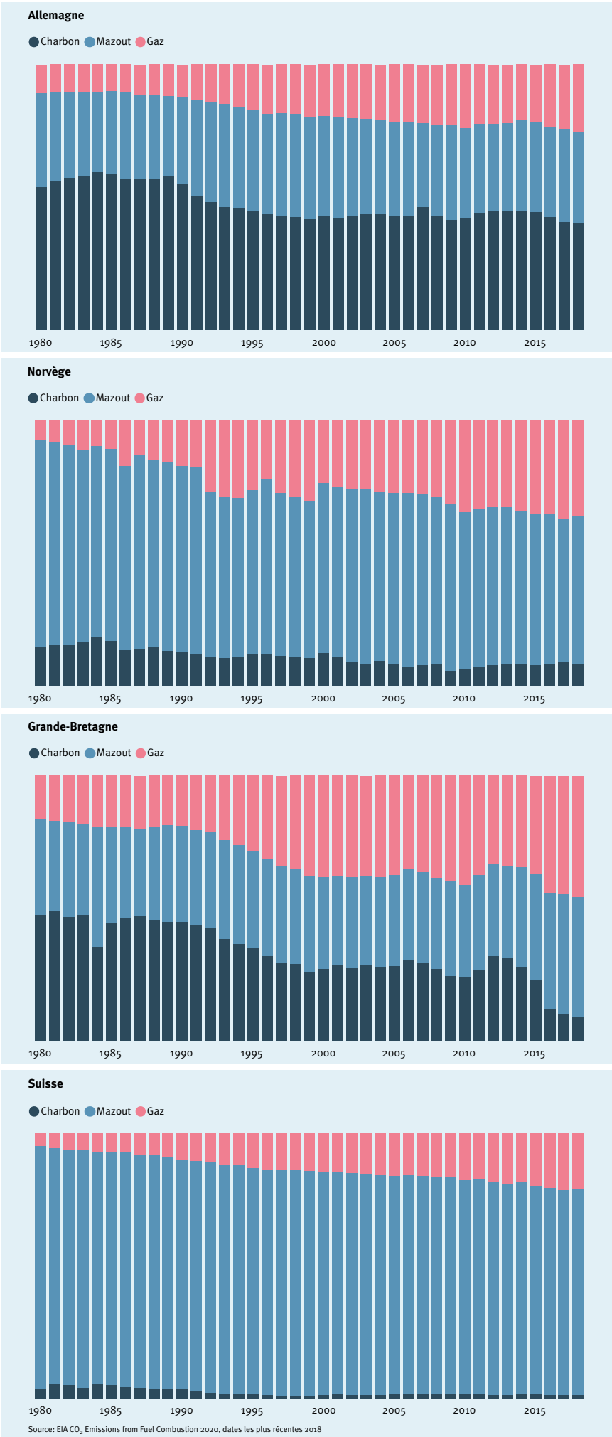
Évolution des émissions par agent énergétique, pourcentage
