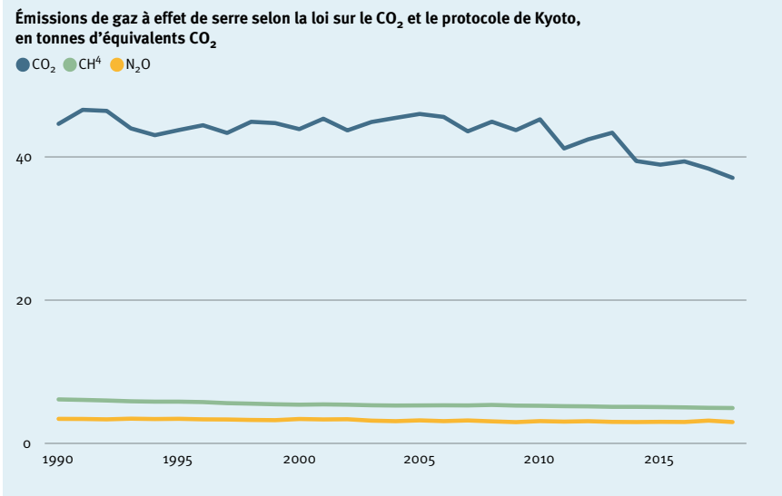
Les émissions anthropiques de gaz à effet de serre de la Suisse diminuent. Absolu en millions de tonnes de CO 2 eq par an
